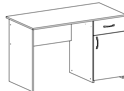
Корпус С-01 в комплекте с фасадами С-013
